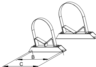
Bild 4: Auflageschellen
